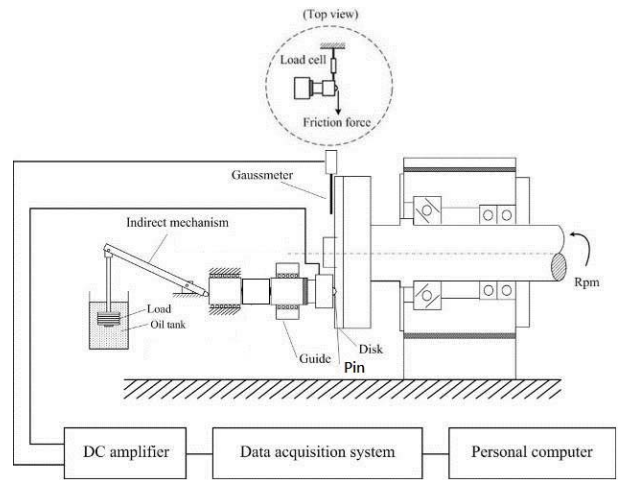
圖 1 旋轉式摩擦磁化試驗機量測系統
