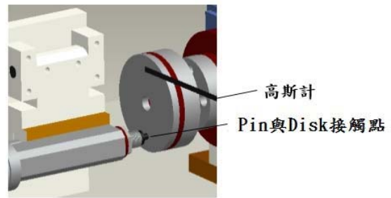
圖 2 試片配置量測之示意圖
